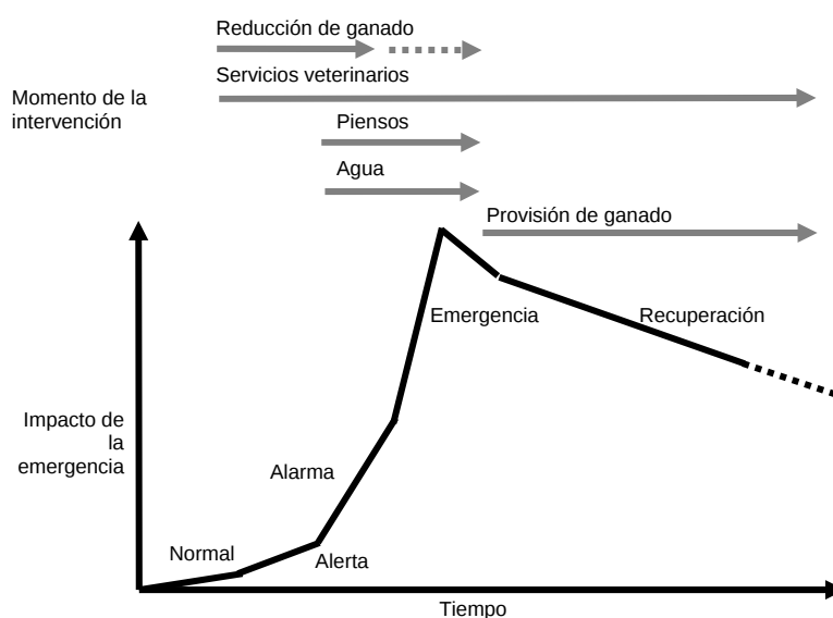
Gráfico 2.2 Caso práctico B: Una sequía en África (de inicio lento)
