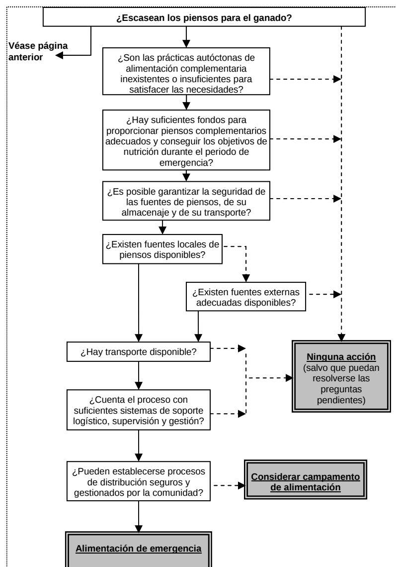
Gráfico 6.1 Árbol de toma de decisiones para las opciones de piensos
