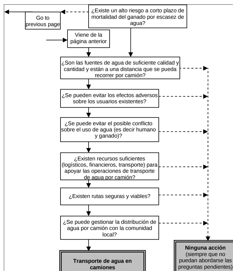
Gráfico 7.1: Árbol de toma de decisiones para las opciones de agua
