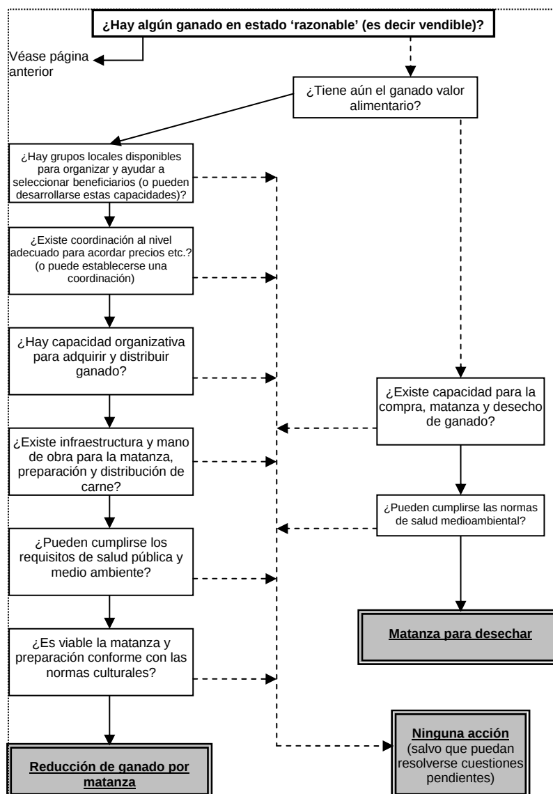
Gráfico 4.1 Árbol de toma de decisiones para las opciones de reducción de ganado
